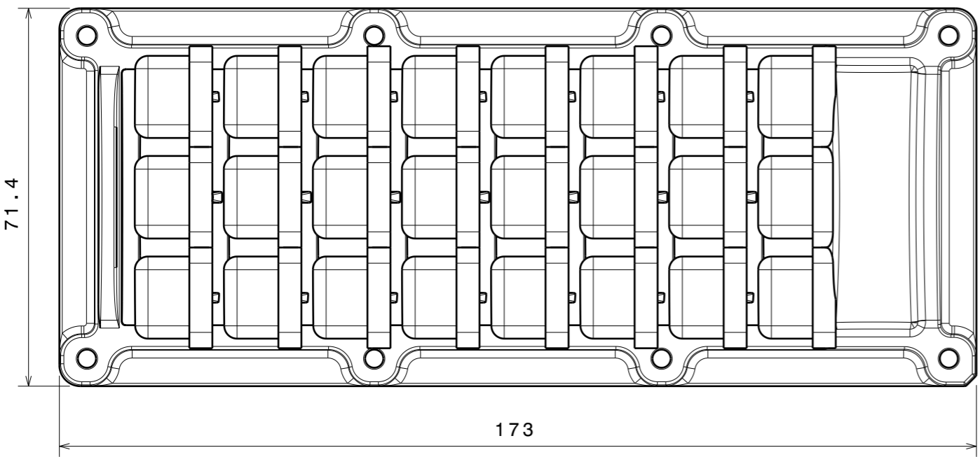
Top view Scale: 1:1
